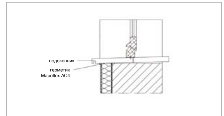
П. 11 – Вертикальный разрез притвора окна
