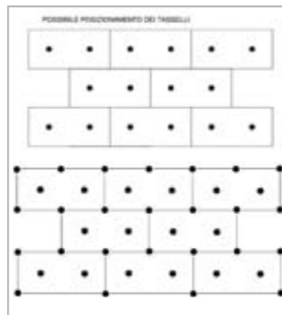
Рис. 5.14 – Расположение дюбелей
