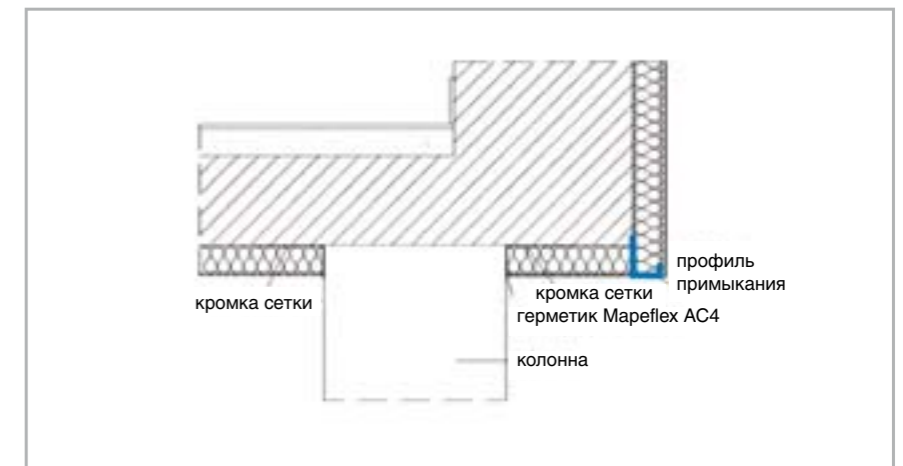
П. 17 – Вертикальный разрез конструкции типа наружной колонны
