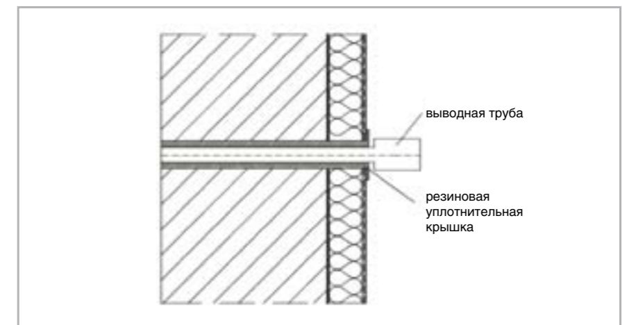
П. 6 – Вертикальный разрез трубы подвода воздуха
