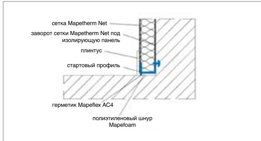
П. 13 – Плинтус на балконе
