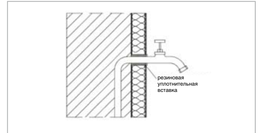
П. 4 – Вертикальный разрез наружной трубы
