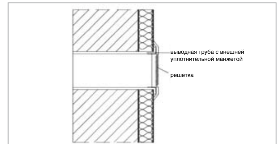
П. 5 – Вертикальный разрез вентиляционного канала
