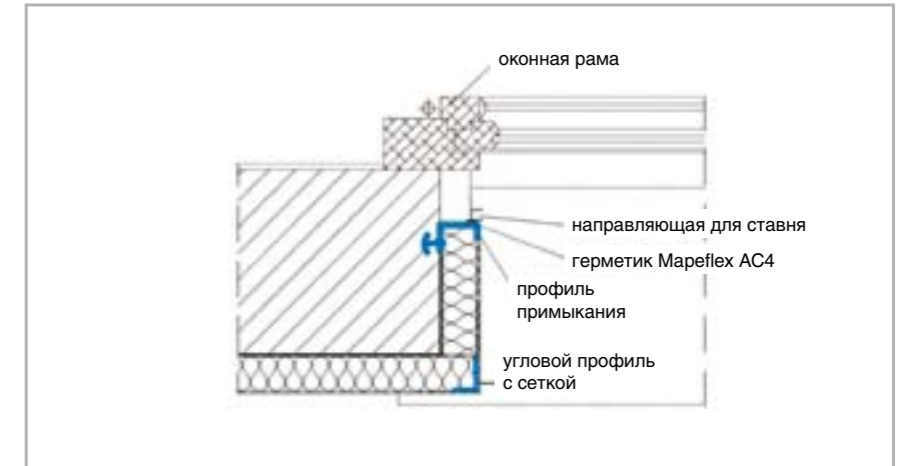
П. 16 – Горизонтальный разрез окна с выступающей роликовой шторкой
