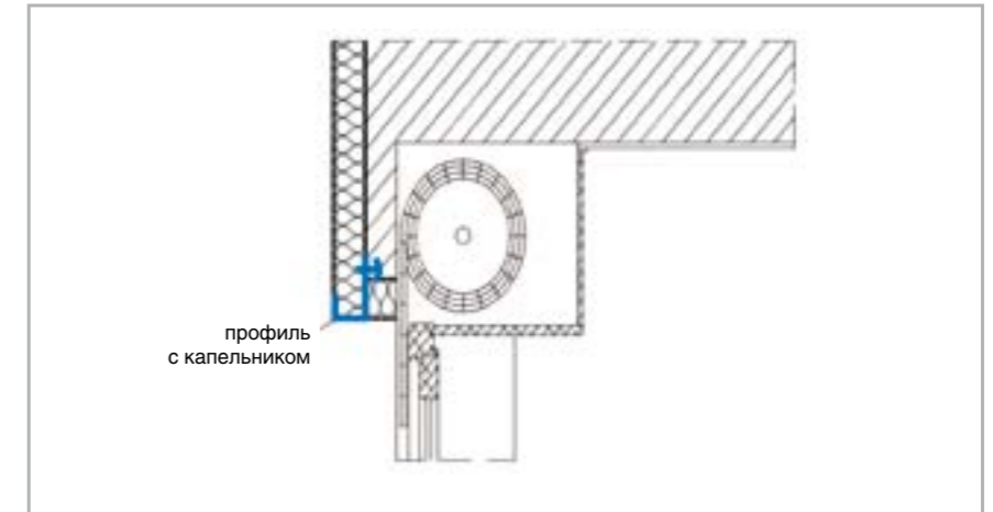
П. 10 – Вертикальный разрез окна с местом для роликовой шторы
