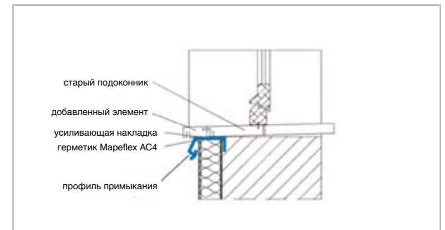
П. 12 – Вертикальный разрез притвора окна с расширением
