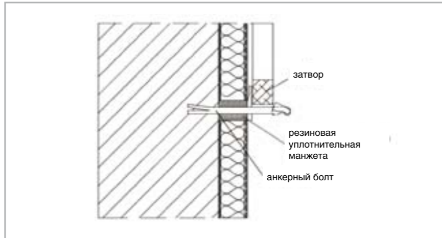
П. 7 – Вертикальный разрез ограничителя роликовой шторы
